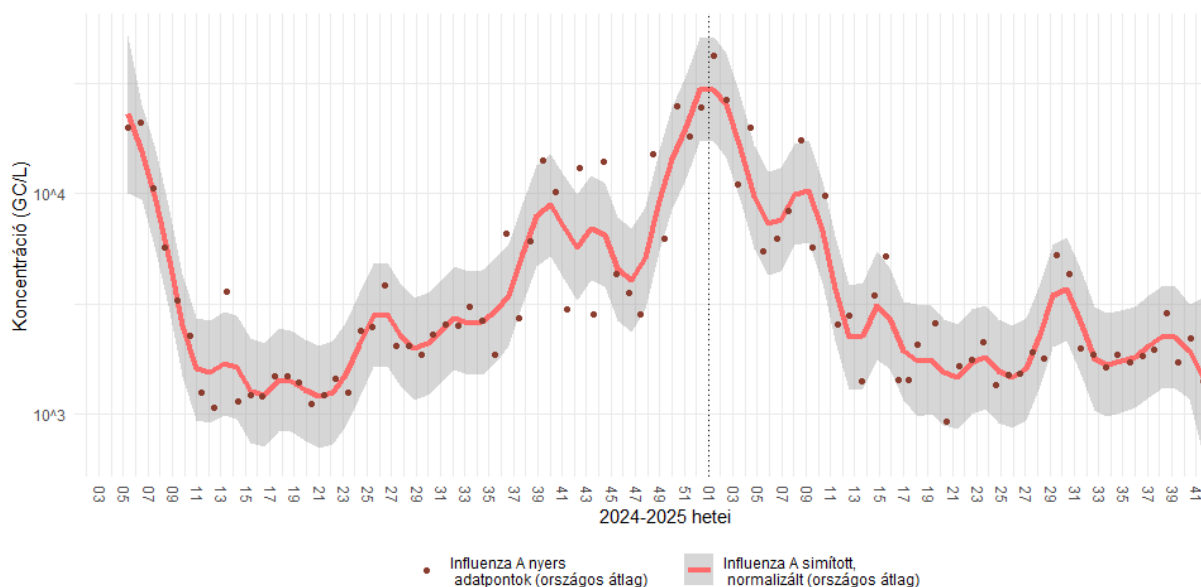
7. ábra A szennyvízben mért Influenza A kópiaszám országos, lakosságarányos súlyozott átlaga. A véletlenszerű ingadozások hatásának kiszűrése érdekében nem-parametrikus regressziós LOWESS (LOcally WEighted Scatter-plot Smoother) módszer felhasználásával létrehozott simított görbe (piros). A narancssárga pontok a nyers adatokat mutatják, a szürke sáv a 95%-os konfidencia-intervallumot jelöli.
