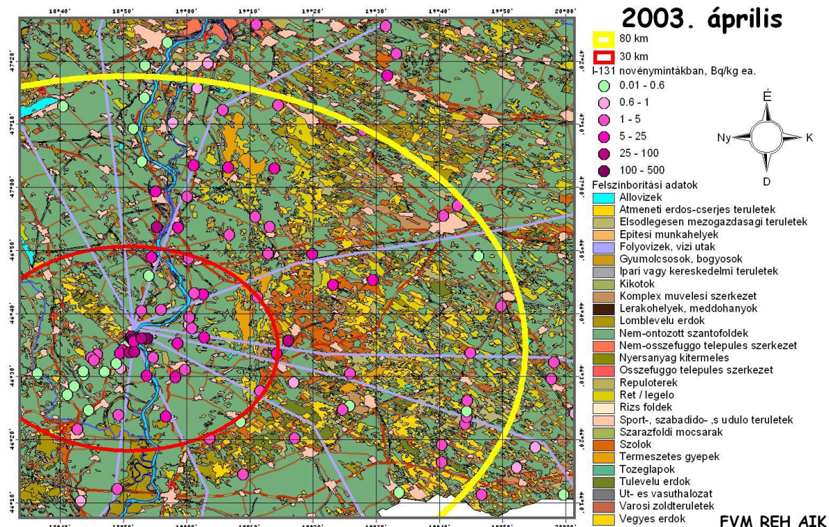
3.4. ábra A növénymintákban mért ^{131}\text{I} aktivitáskonzentrációk (eredeti anyagra)
