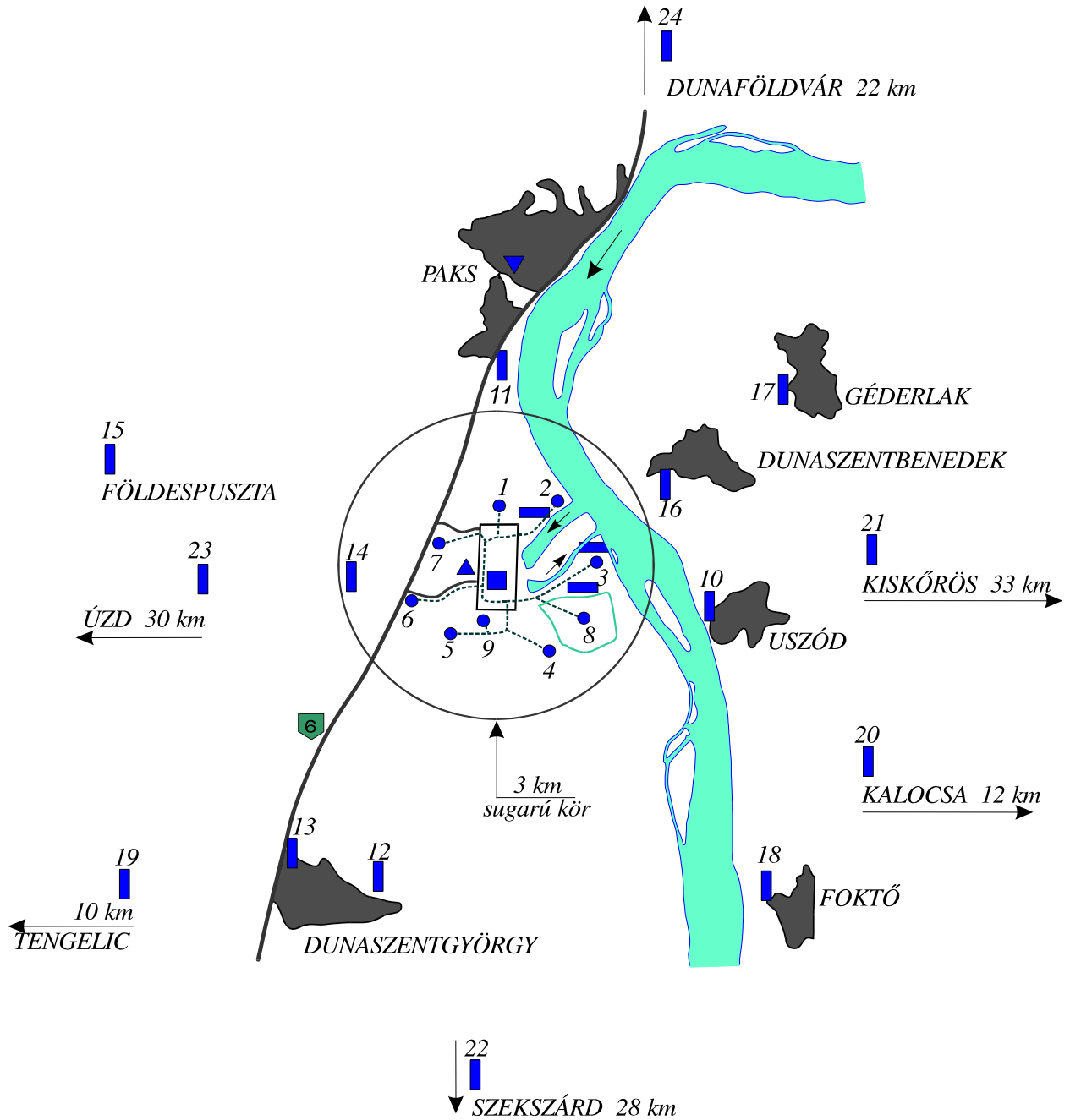
A Paksi Atomerőmű üzemi környezetellenőrző állomáshálózata
