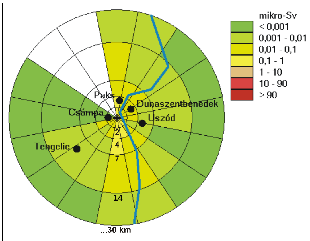
4.1. ábra A radiojód és nemesgáz izotópoktól származó teljes sugárterhelés szektoronkénti megoszlása
